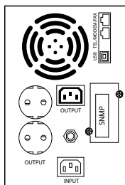
Задняя панель напольного ИБП 1000-2000 ВА
